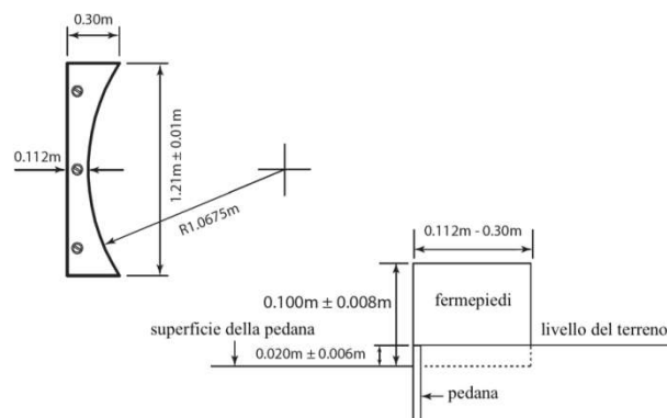
Figura RT 32 a – Pianta del fermapièdi (vista dall'alto e laterale)
