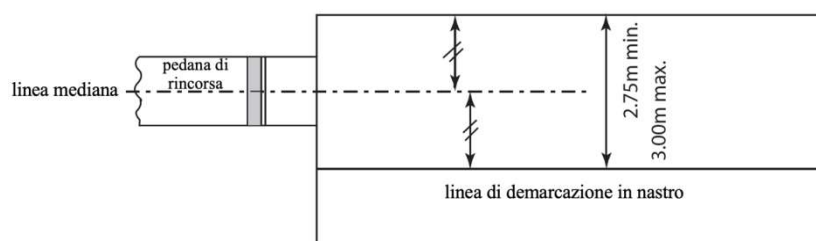
Figura RT 29 b – Zona di caduta per Salto in Lungo e Salto Triplo
