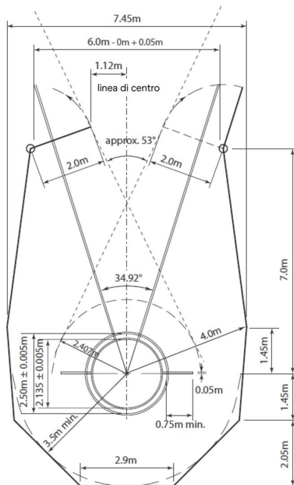
Figura RT 37 a – Gabbia per il Lancio del Martello e del Disco con pedane concentriche (configurazione Lancio del Martello, per lanciaatore destrimano)
